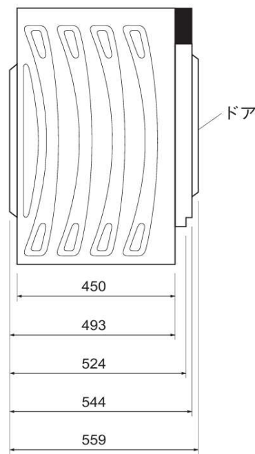
側面図
