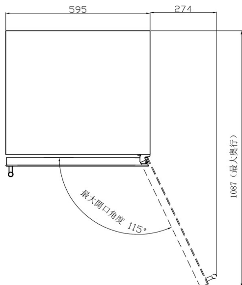
平面図
