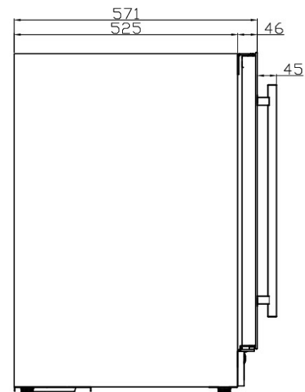
側面図
