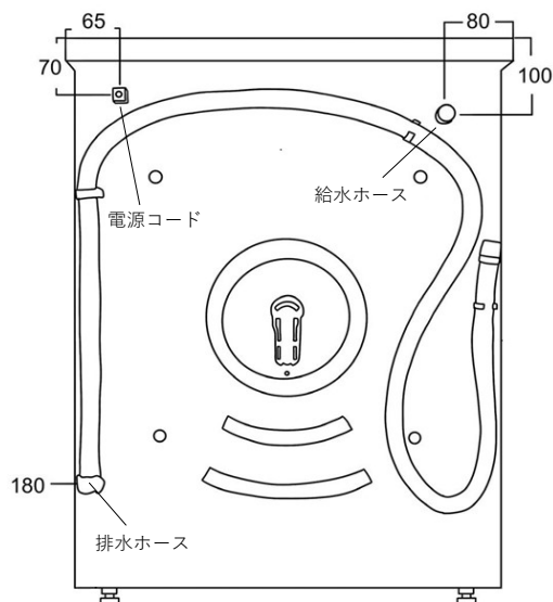
背面図
