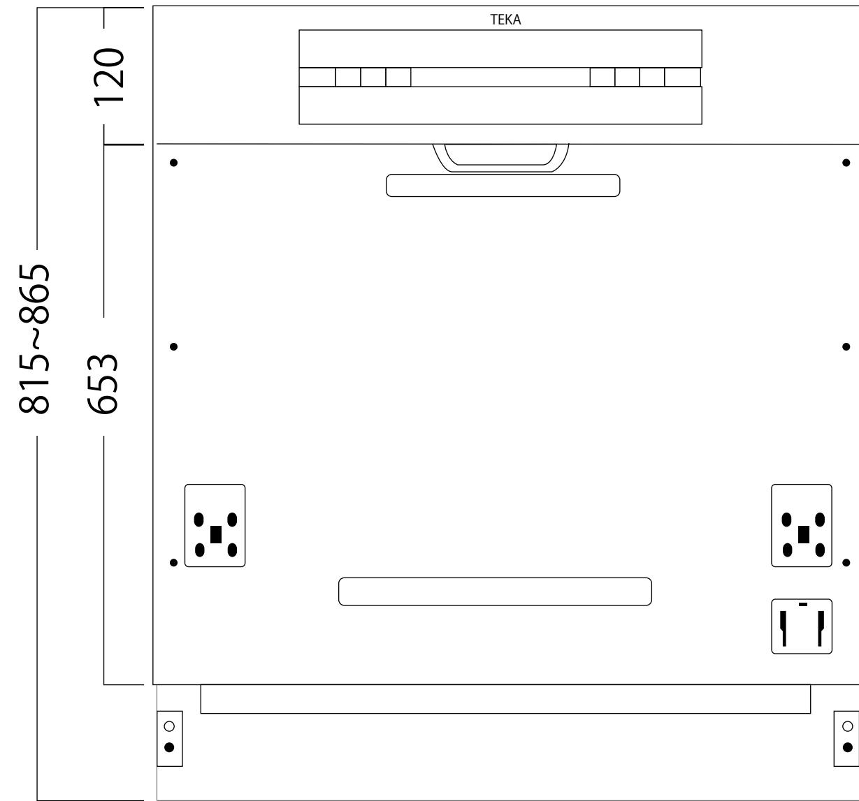
正面図
